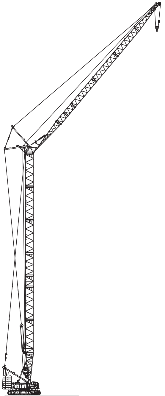
タワー仕様 タワー+タワージブ最長
